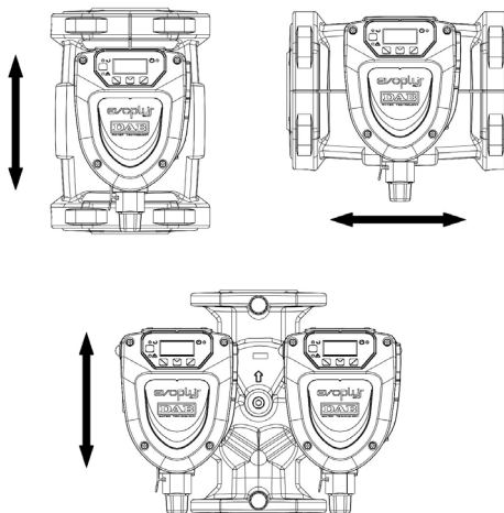
Afbeelding 1: montagepositie
