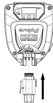
Figure 4 : Connexion connecteur d'alimentation
