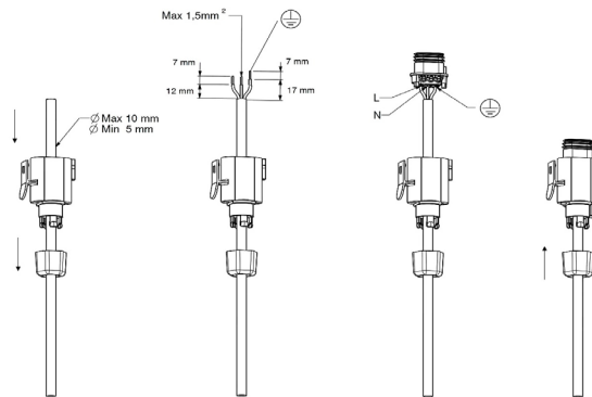
Afbeelding 3: Bedrading voedingsstekker
